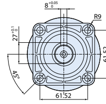
Flangiatura pompa Pump flange
