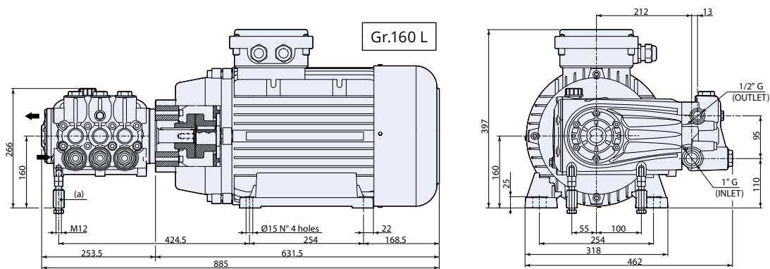
Motore elettrico GR. 160L con giunto flessibile interno. GR. 160L electric motor with internal flexible joint.
